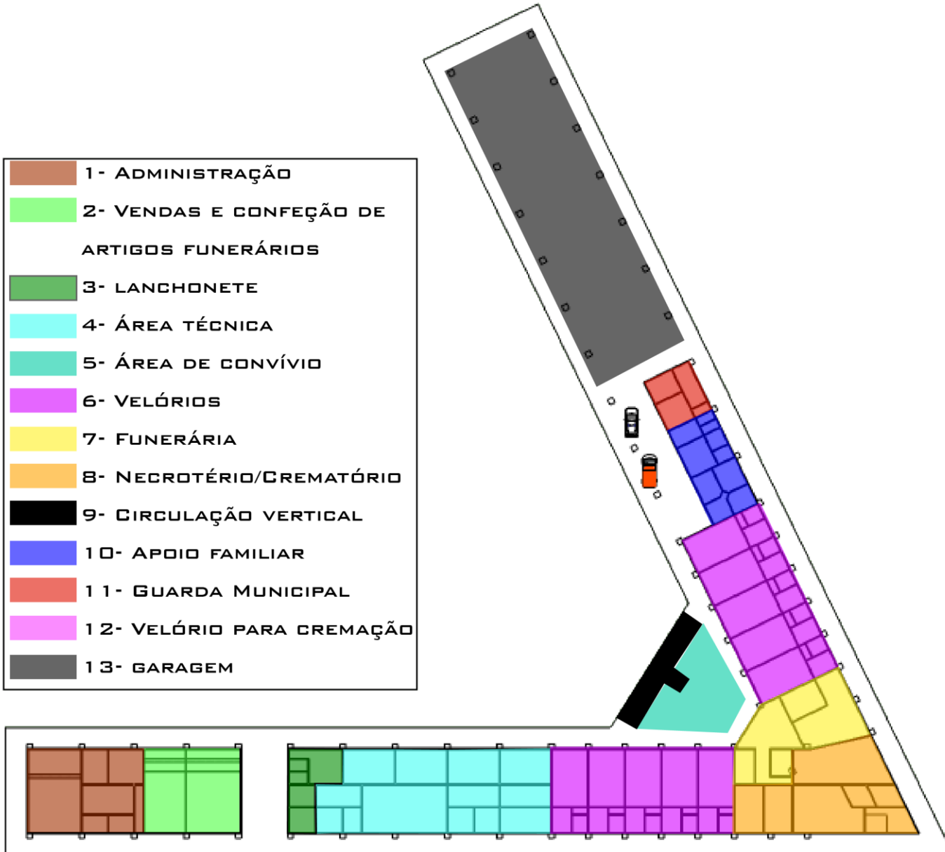
PLANTA - TÉRREO
